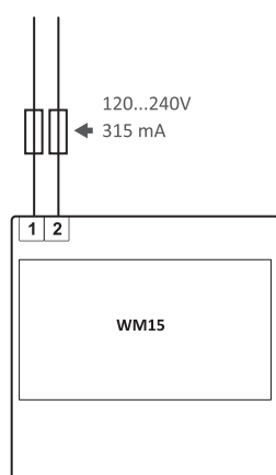
Abb. 12 Hilfsstromversorgung (H)
