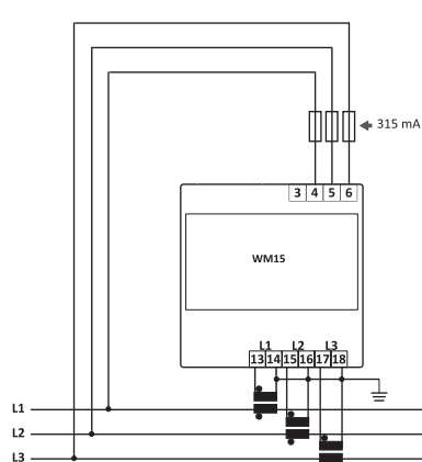
Abb. 10 Dreiphasig ohne Nullleiter (3-drahtig)
