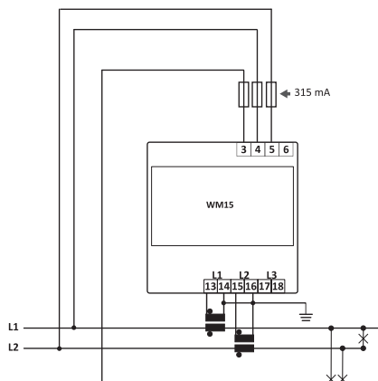
Abb. 8 Zweiphasen-System mit Nullleiter (3 Adern)
