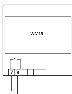
Abb. 13 Digitalausgang
