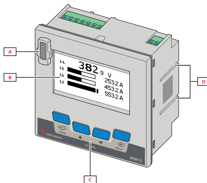
Abb. 1 Vorderseite
