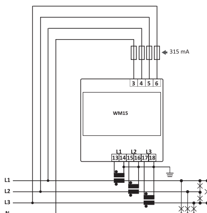
Abb. 6 Dreiphasig mit Nullleiter (4-drahtig)
