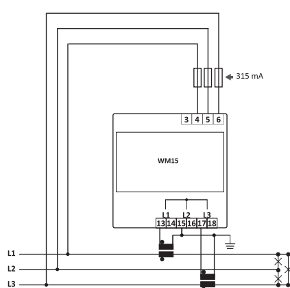
Abb. 7 Dreiphasig ohne Nullleiter (3-drahtig)
