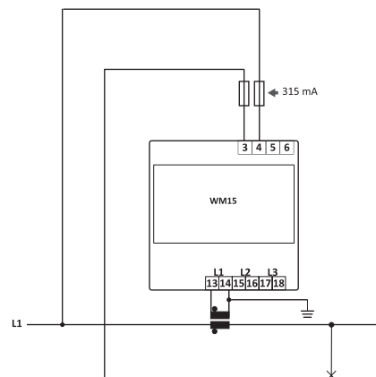
Abb. 9 Einphasig (2-drahtig)
