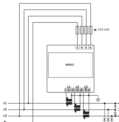
Abb. 11 Dreiphasig mit Nullleiter (4-drahtig)
