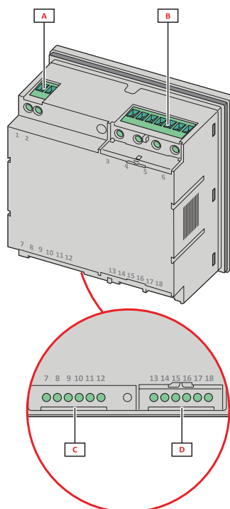
Abb. 2 Rückseite
